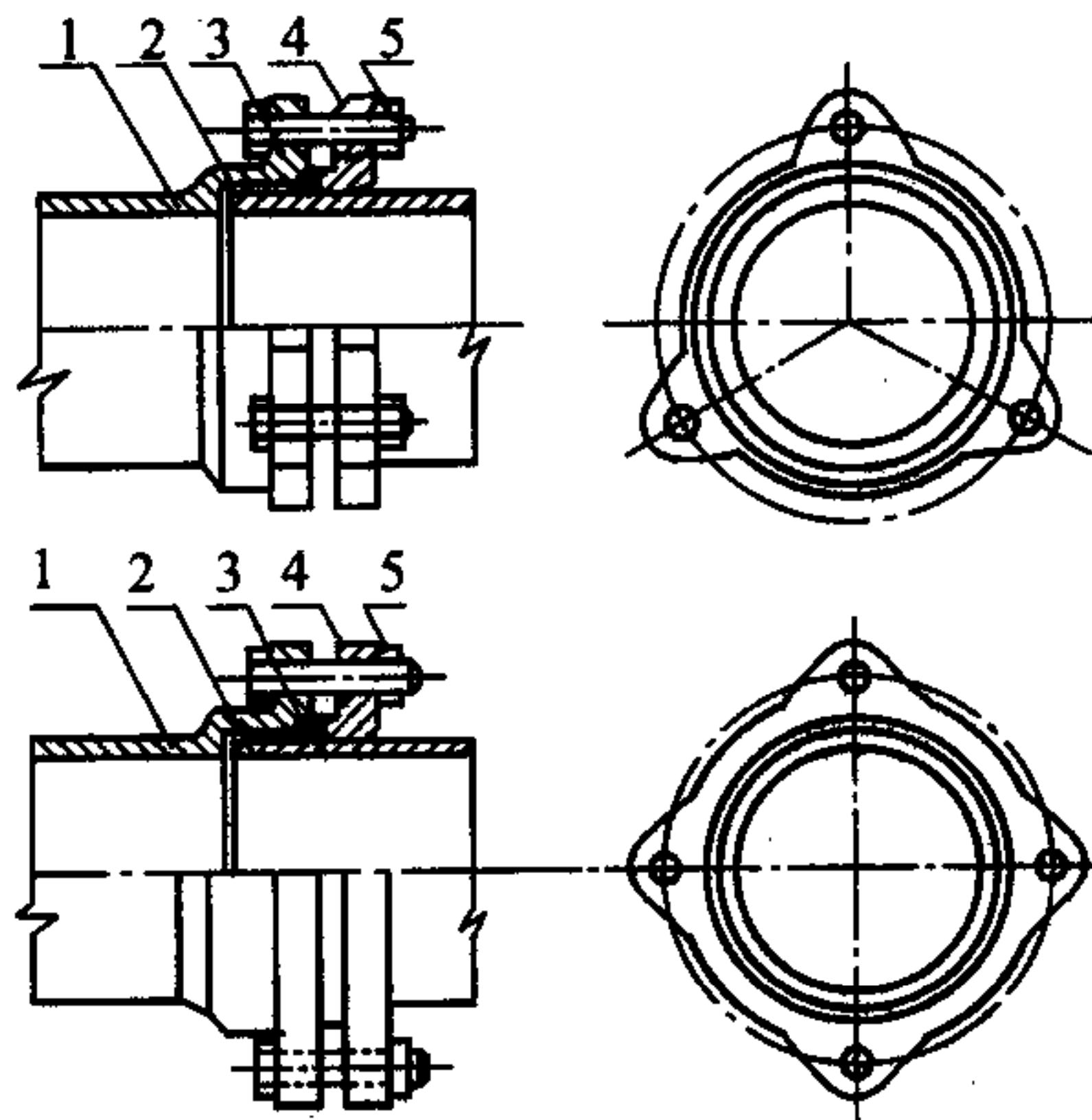
图2 铸铁管法兰机械式接口连接示意图
