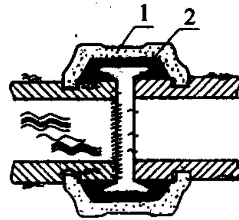
图3 钢管沟槽式连接示意图
