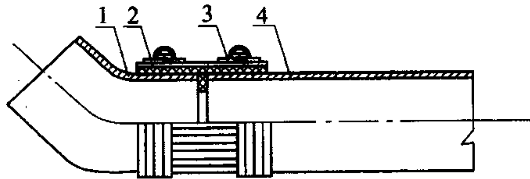
图1 铸铁管卡箍式接口连接示意图
